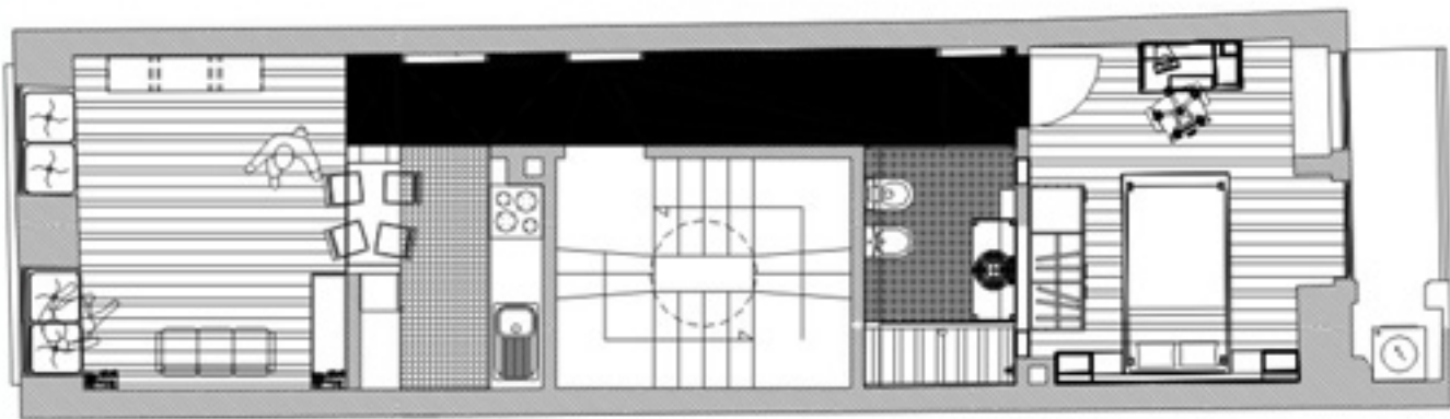
Planta 1º Andar
